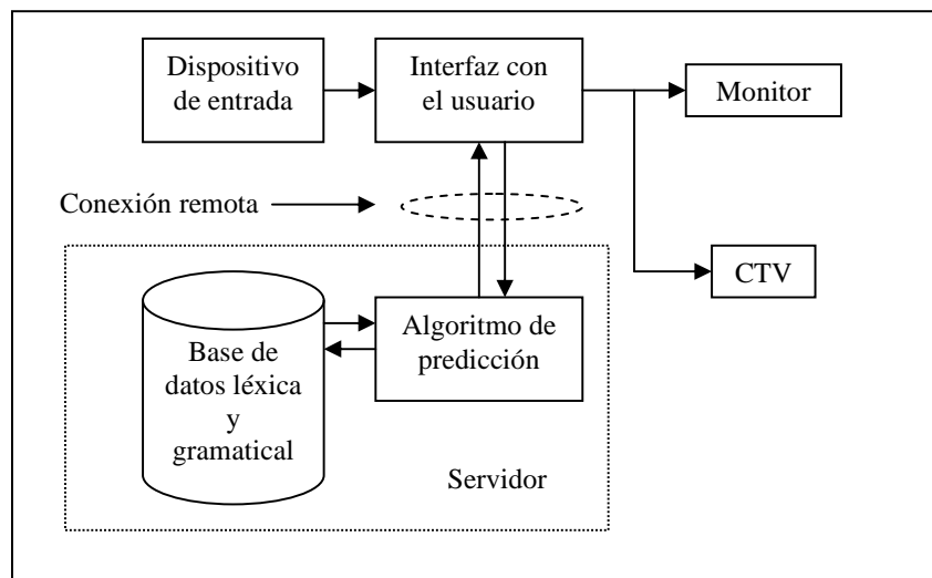
Figura 2: Esquema del sistema cliente/servidor Casandra para el apoyo a la escritura por predicción de palabras.
